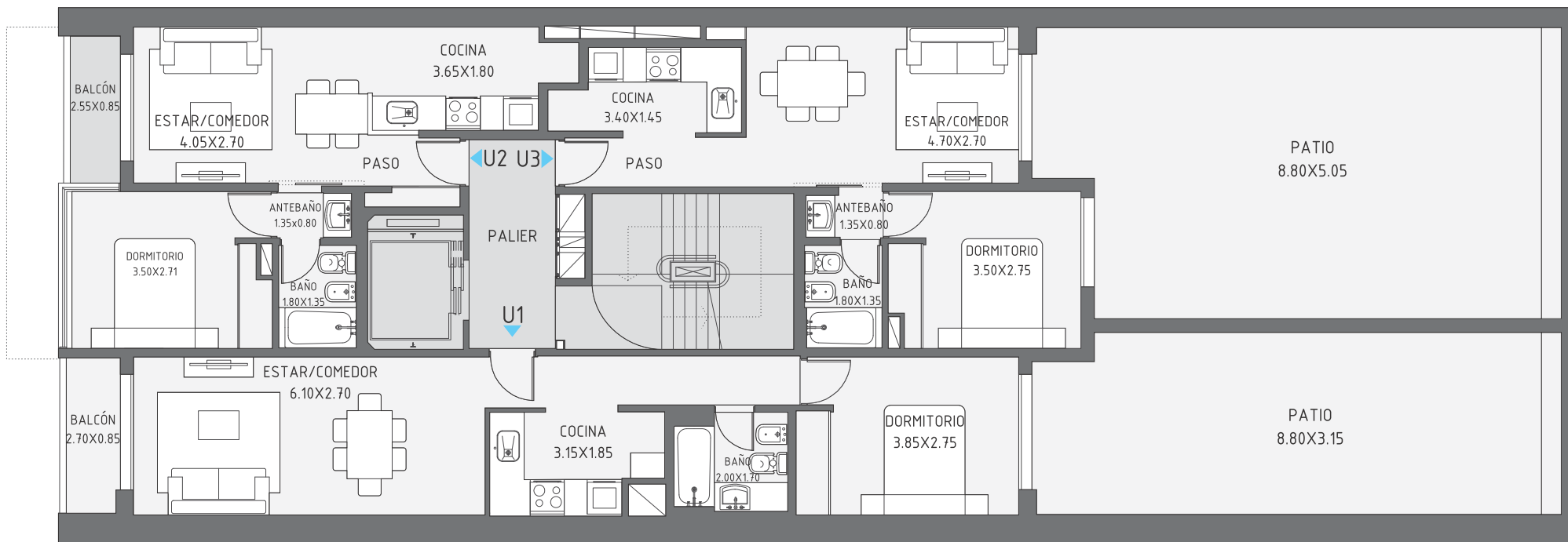
PLANTA PISO 1°
