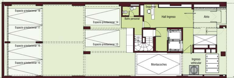
PLANTA INGRESO
