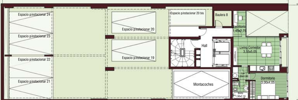
PLANTA 1º PISO
