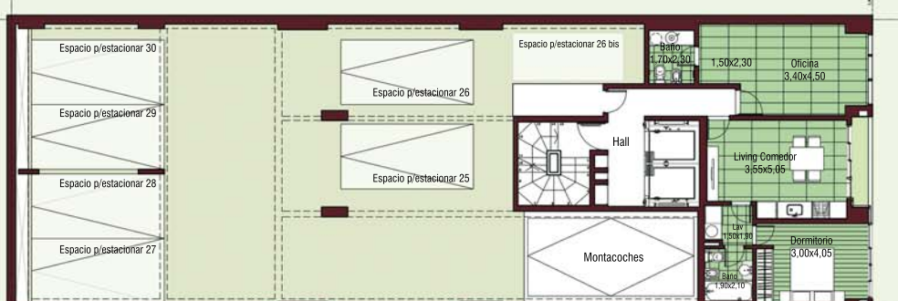
PLANTA 2º PISO
