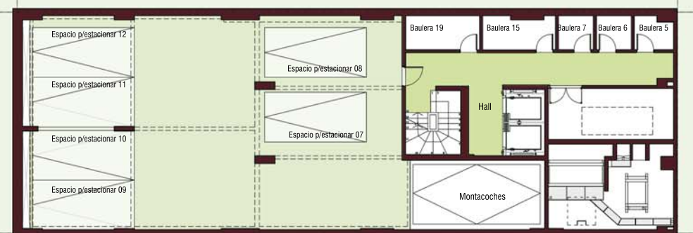
PLANTA 1º SUBSUELO
