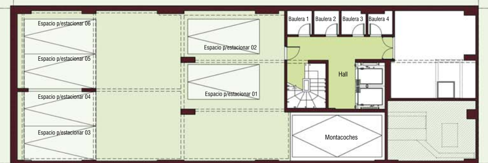
PLANTA 2º SUBSUELO
